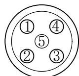
公针芯焊接端 焊接端排序图
