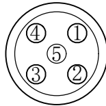
母针芯焊接端 焊接端排序图
