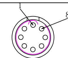
公针芯焊接端 焊接排序图
