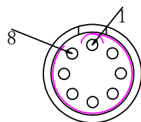
母针芯焊接端 焊接排序图
