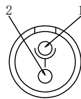
母针芯焊接端 焊接排序图
