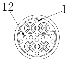
公针芯焊接端 焊接排序图
